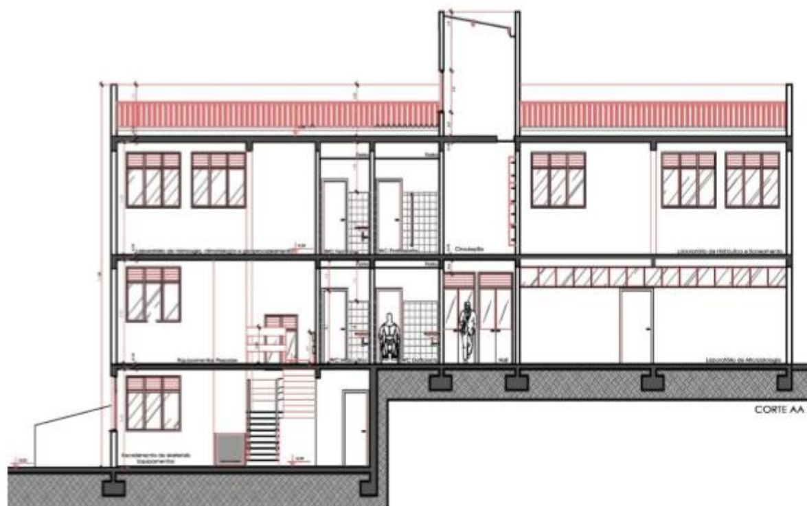
Figura 4 - Corte A da edificação dimensionada
